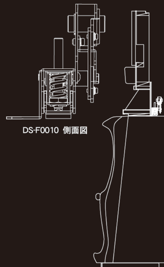
DS-F0010 本体・スロット取付側面図
